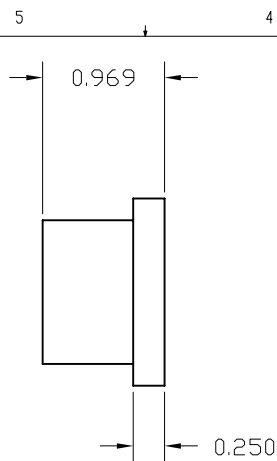
LEFT SIDE
